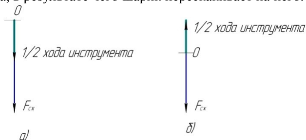
Рисунок 3 – Система сил
