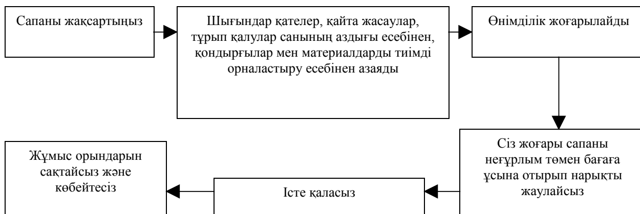
Сурет 1 – Демингтің тізбекті реакциясы
