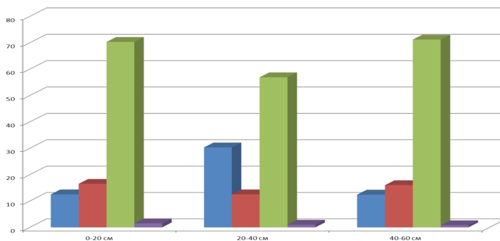
Рисунок 4 – Содержание тяжёлых металлов на супераквальном ландшафте Петровского колочного леса, в %
